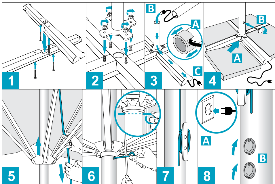
Obrázek 2. Průběh montáže
