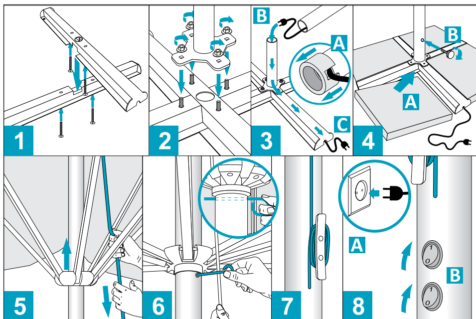
Obrázok 2. Priebeh montáže
