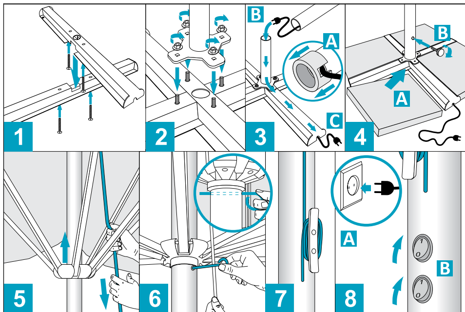
Rys. 2. Przebieg montażu
