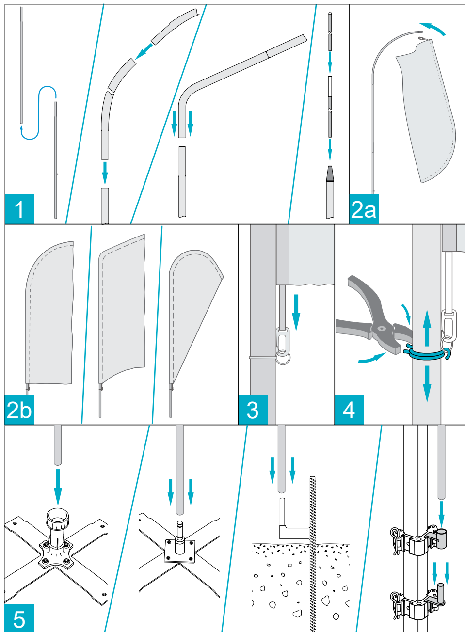
Rys. 5. Przebieg montażu
